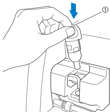
① Poignée
