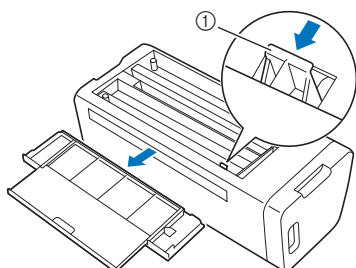
① Levier de déverrouillage du plateau arrière
