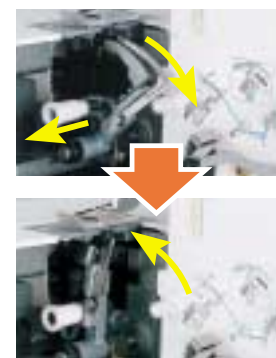
Enfilage rapide du boucleur inférieur
